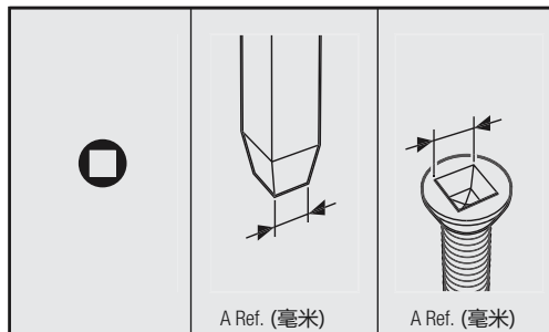
四方螺丝
