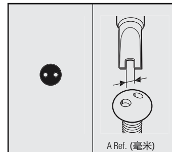
双控螺丝
